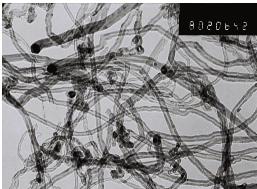
TEM
