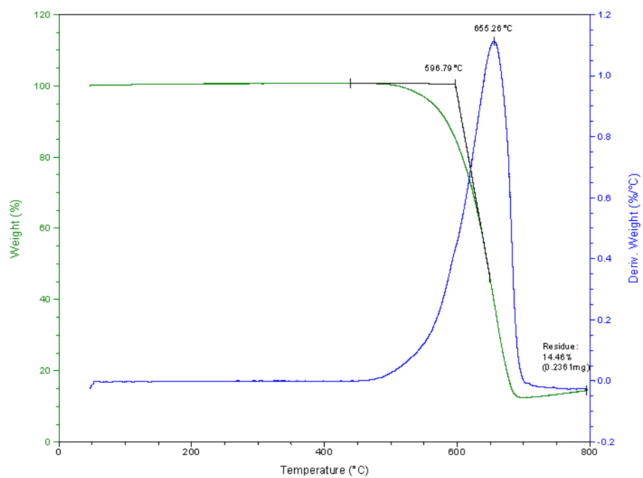
TGA
